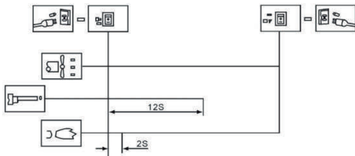
рис. 8. Схема зажигания
